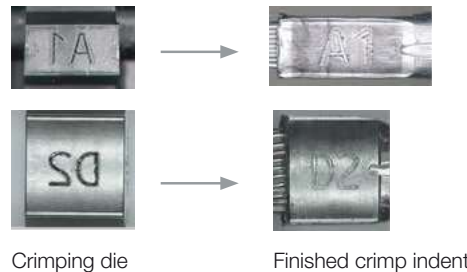
Crimping die
